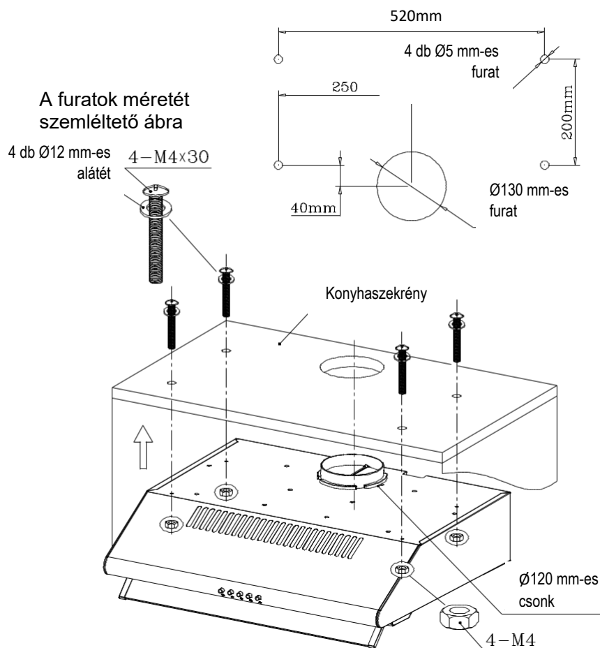
Beépítési rajz
