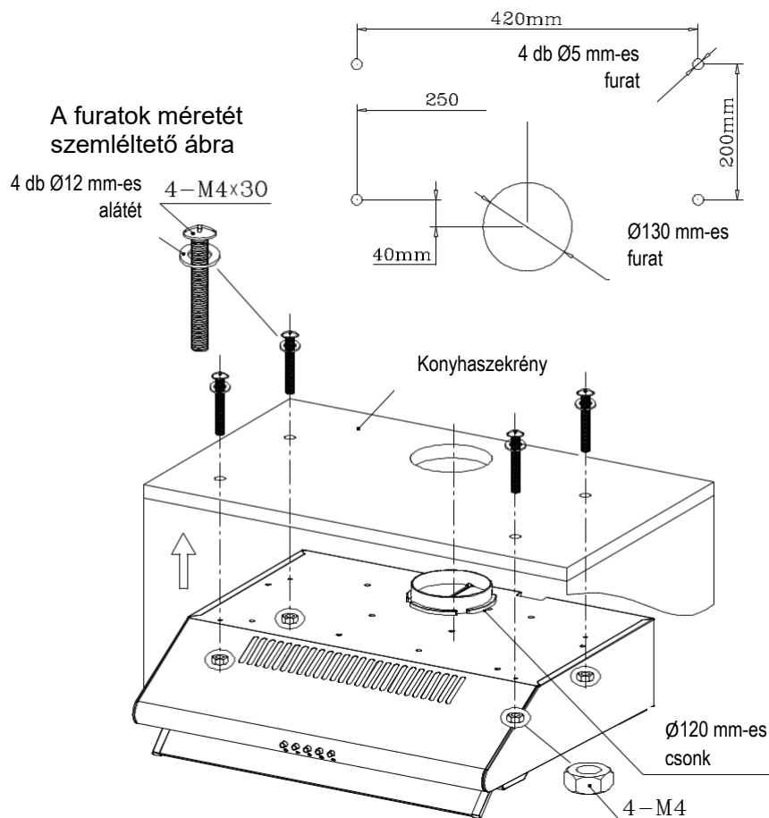
Beépítési rajz
