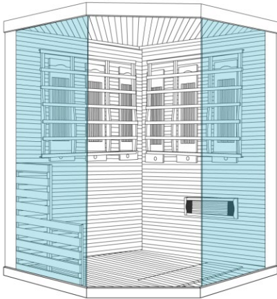
(5) A 4*40 csavarok segítségével rögzítse az ülőkék bal oldali tartóelemét.
